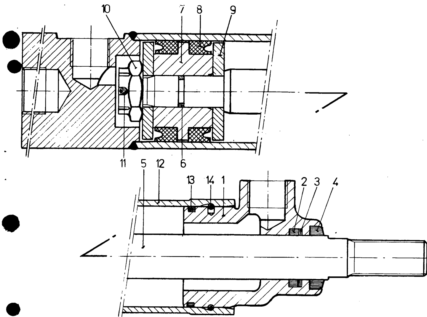
CILINDER VOOR VOLHYDRAULISCH STUUR CYLINDER FOR POWER STEERING VERIN POUR DIRECTION ASSISTEE ARBEITSZYLINDER FÜR HYDRAULISCHE LENKUNG
