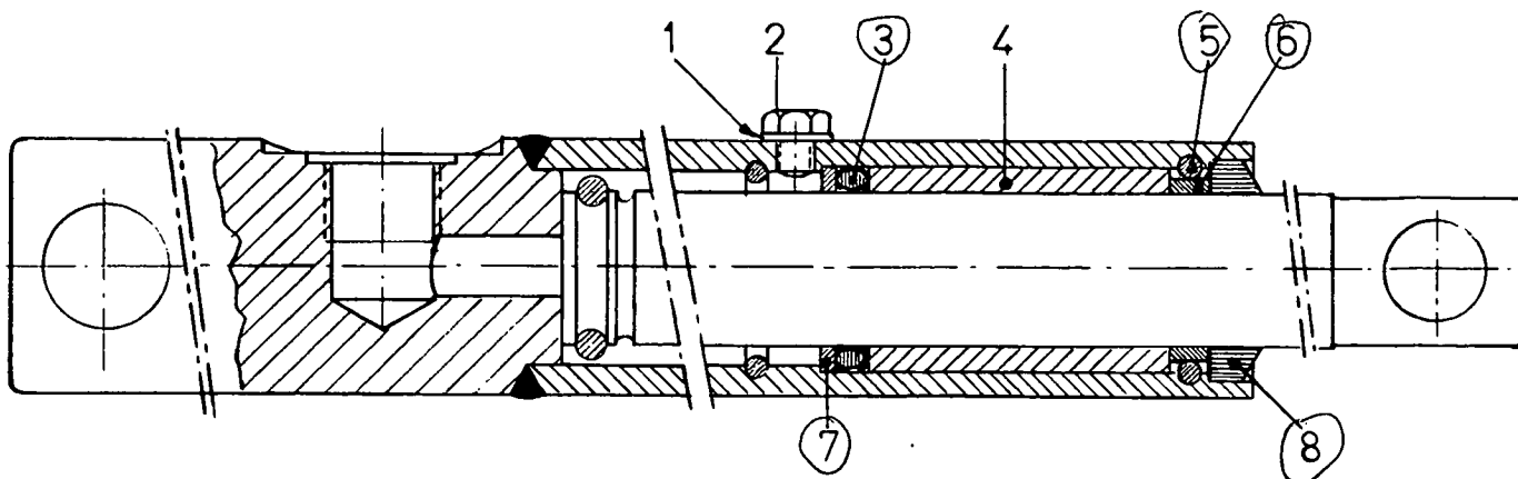
HEFCILINDER - CYLINDER - VERIN - ARBEITSZYLINDER 330893
