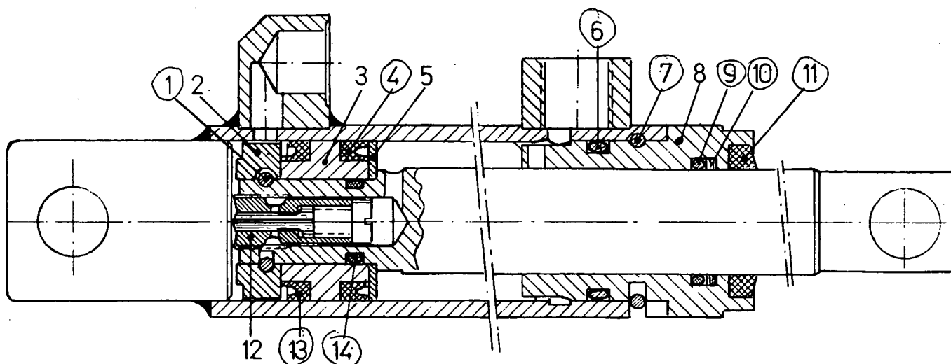
HEFCILINDER - CYLINDER - VERIN - ARBEITSZYLINDER 330892
